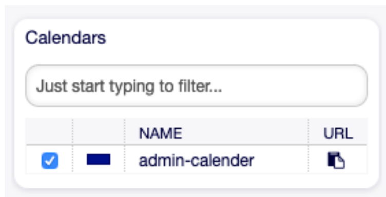
Fig. 5.3: Calendars Widget
